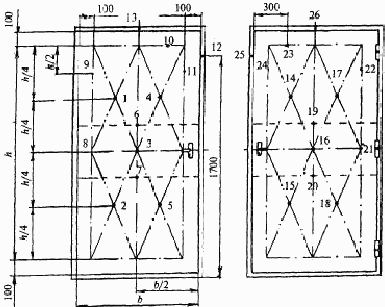
Рисунок 1 — Схема установки термоэлектрических преобразователей (термопар) на несобогреваемой поверхности однопольных дверей
